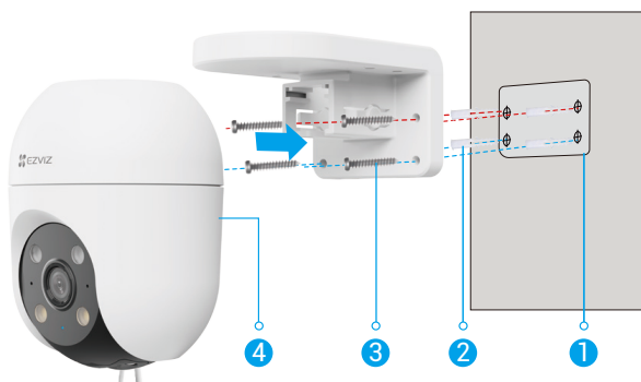
Fig. 2 Montagem na parede
