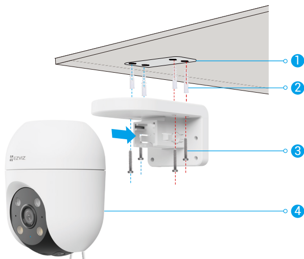
Fig. 1 Montagem no teto
